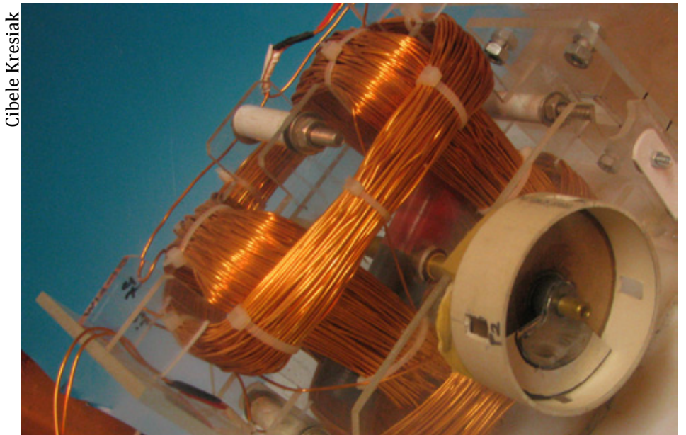
Acima, protótipo funcional do Keppe Motor
